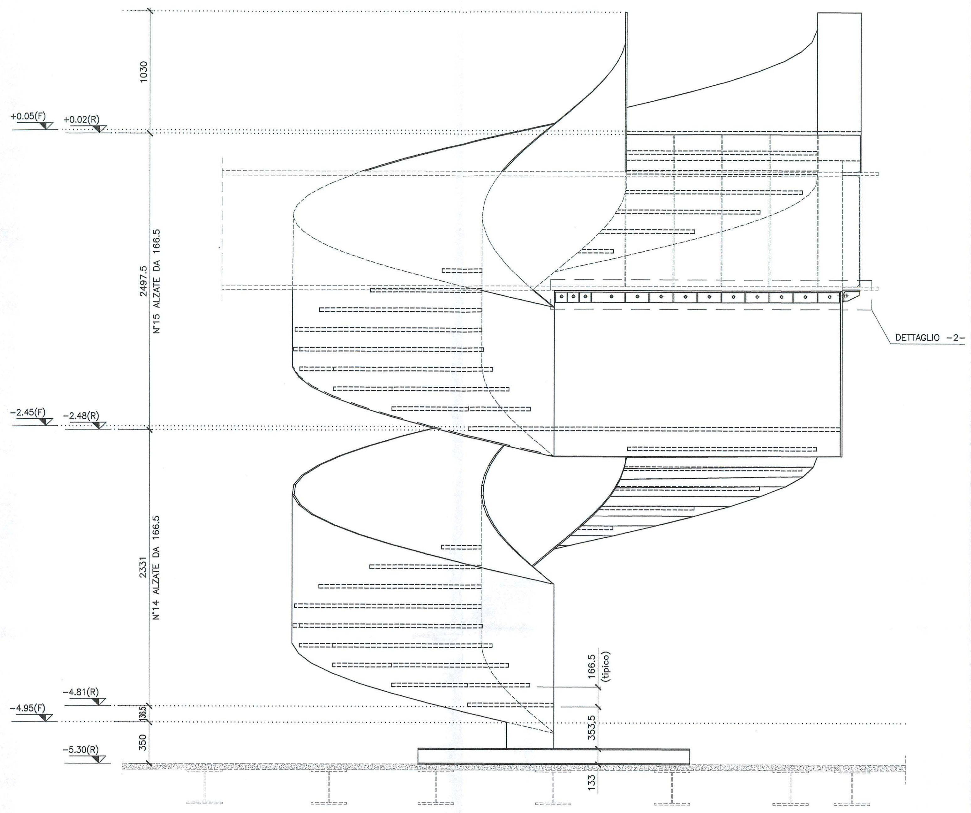
VISTA -1- RAPP. 1:20
