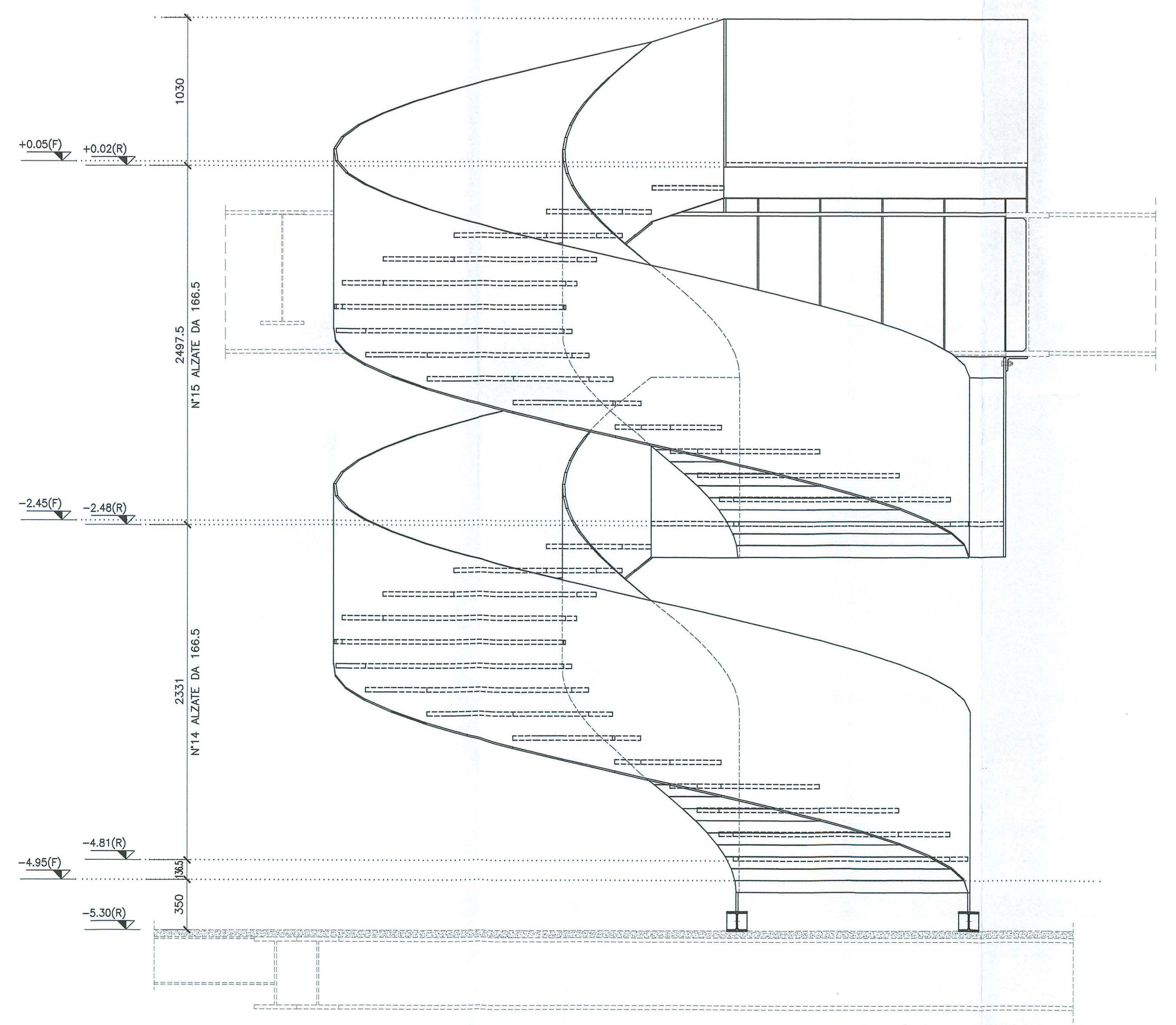
VISTA -4- RAPP. 1:20
