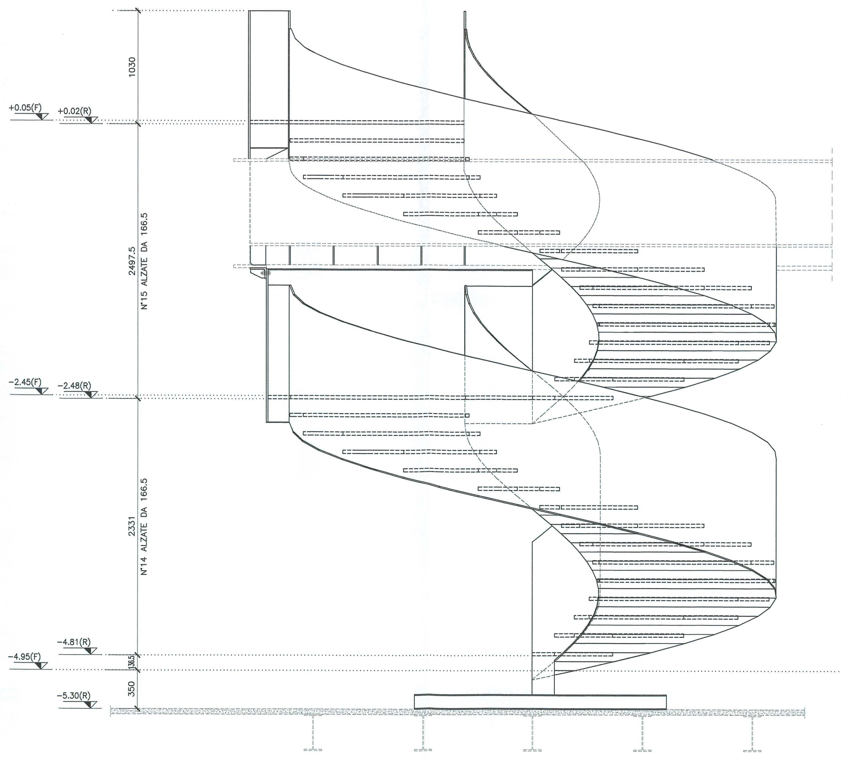
VISTA -3- RAPP. 1:20
