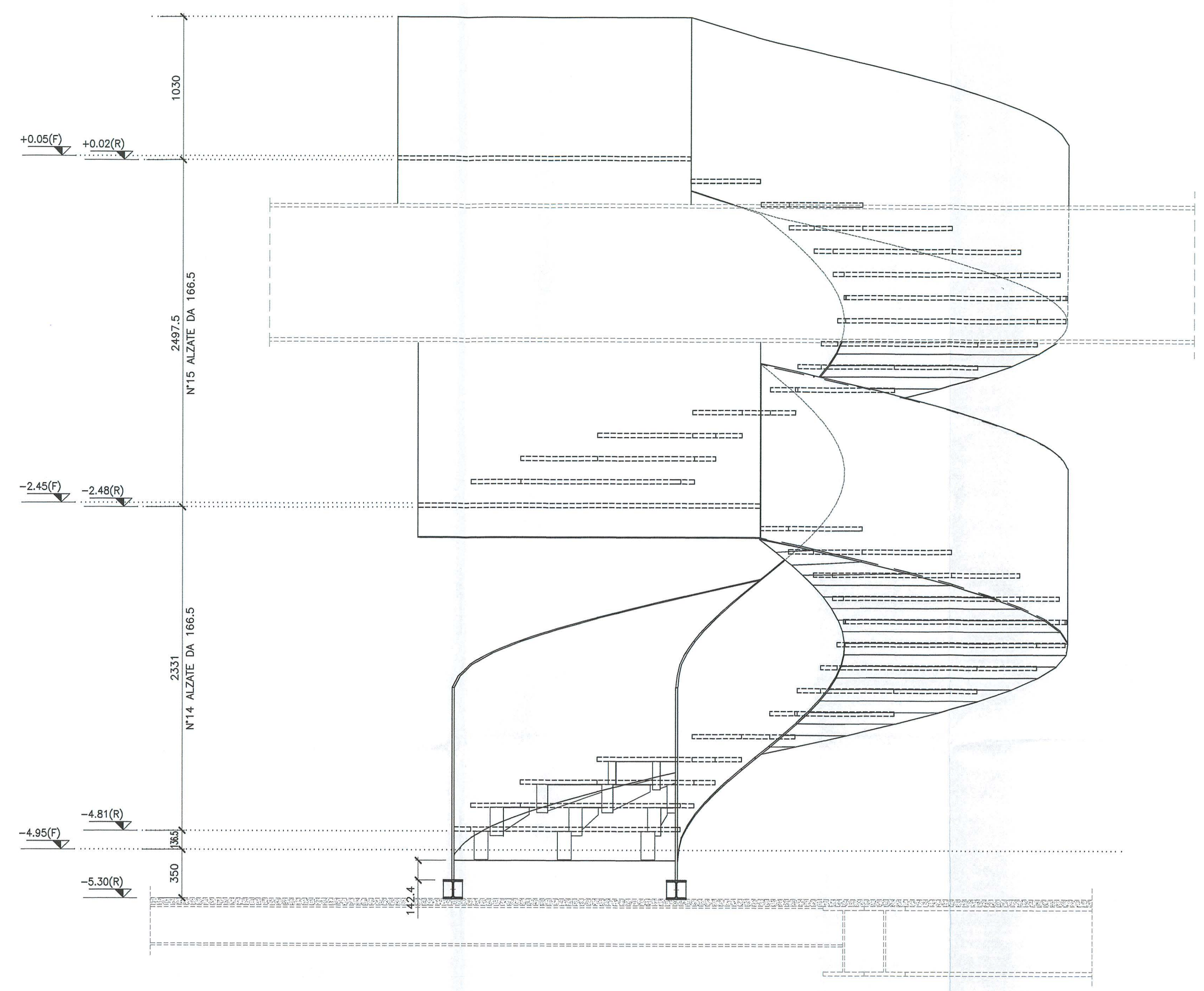
VISTA -2- RAPP. 1:20
